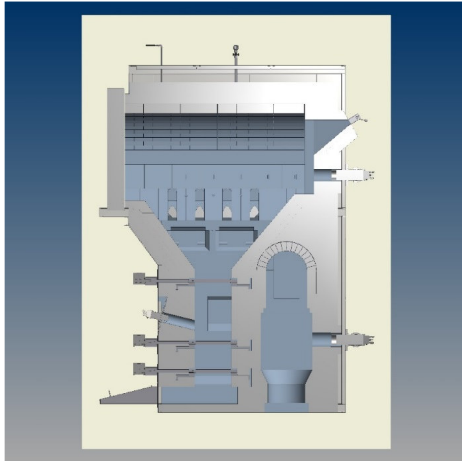
Etagenofen (Graphik: IFZW GmbH)
