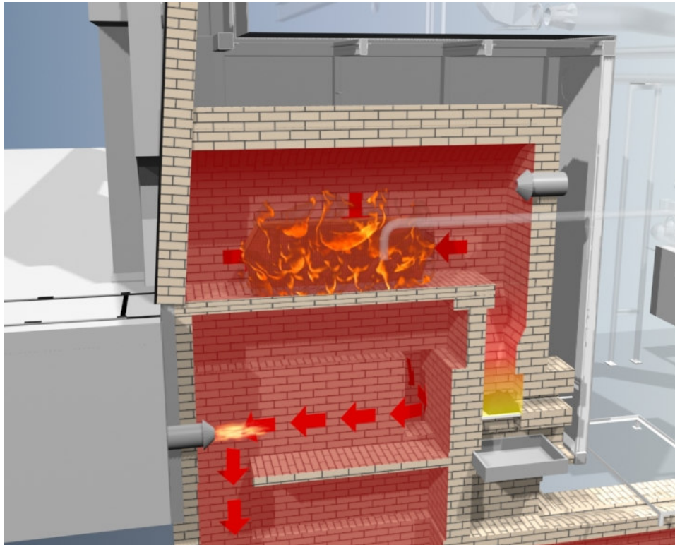
Flachbettofen (Graphik: Heinicke GmbH)
